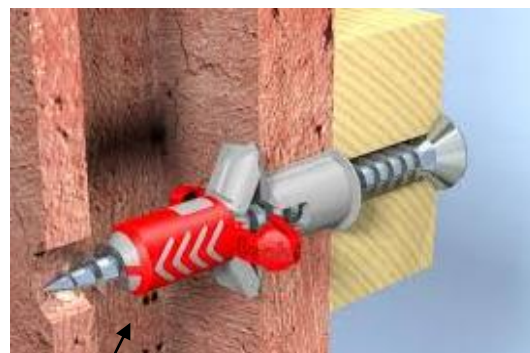
Ukážky rozpnutia a utesnenia dvoch komponentov hmoždiny
